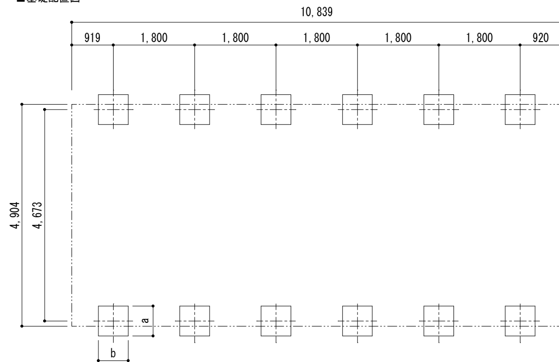
■基礎配置図
